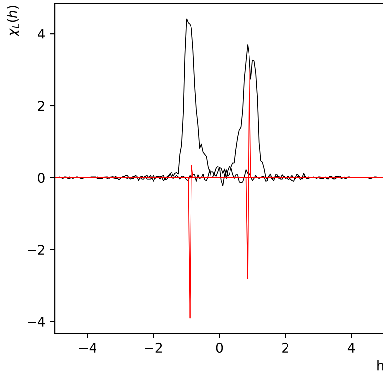
\chi_L(h) réseau de taille L=32 à T=2.0
