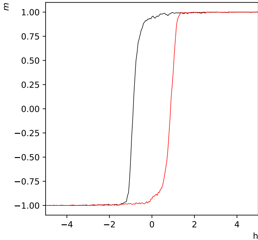
Hystérésis de l'aimantation réseau de taille L=32 - h=5 à T=2.0
